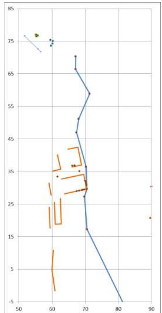
Figur UJ7: Dietrichsens plantegning satt sammen med oppmålingsresultater (2018). Koordinater er EUREF 89 med utgangspunkt i Ø 590800; N 6443900. Punktene i nord er steinsmursegmenter. Den tynne blå linjen er gelenderen langs turstien
