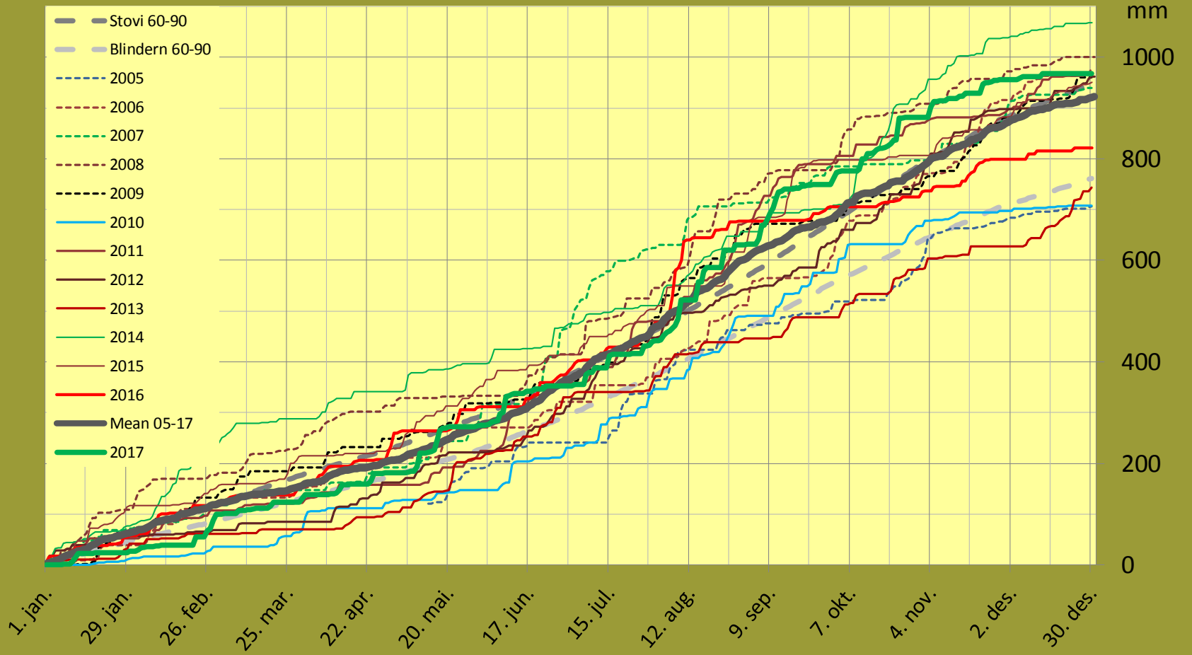
Nedbør Lysejordet 2005 - 2016
